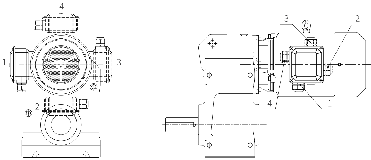
马达接线盒和进线孔位置(视角:马达尾部)
