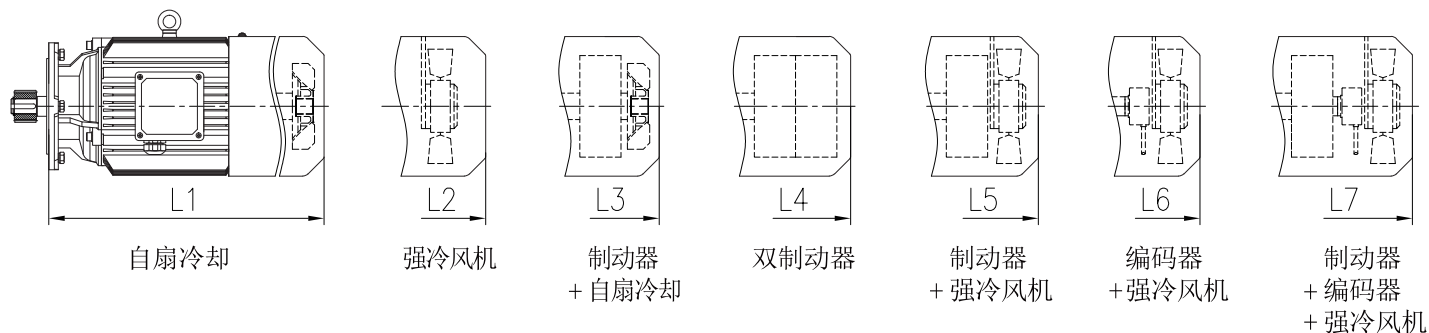
直联马达尺寸表
