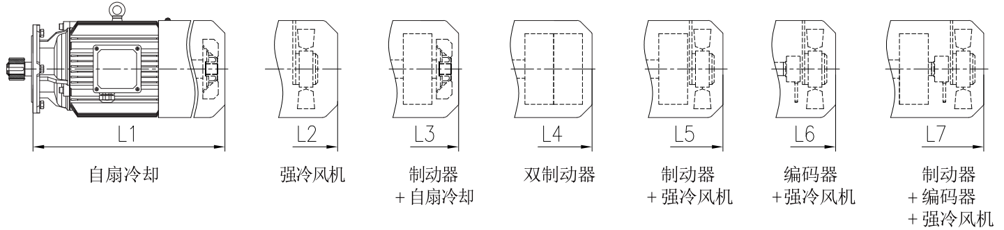
直联马达尺寸表
