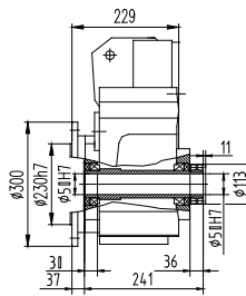
F207FI/F307FI
