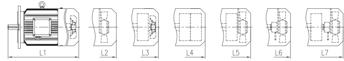
MU马达长度尺寸和重量
