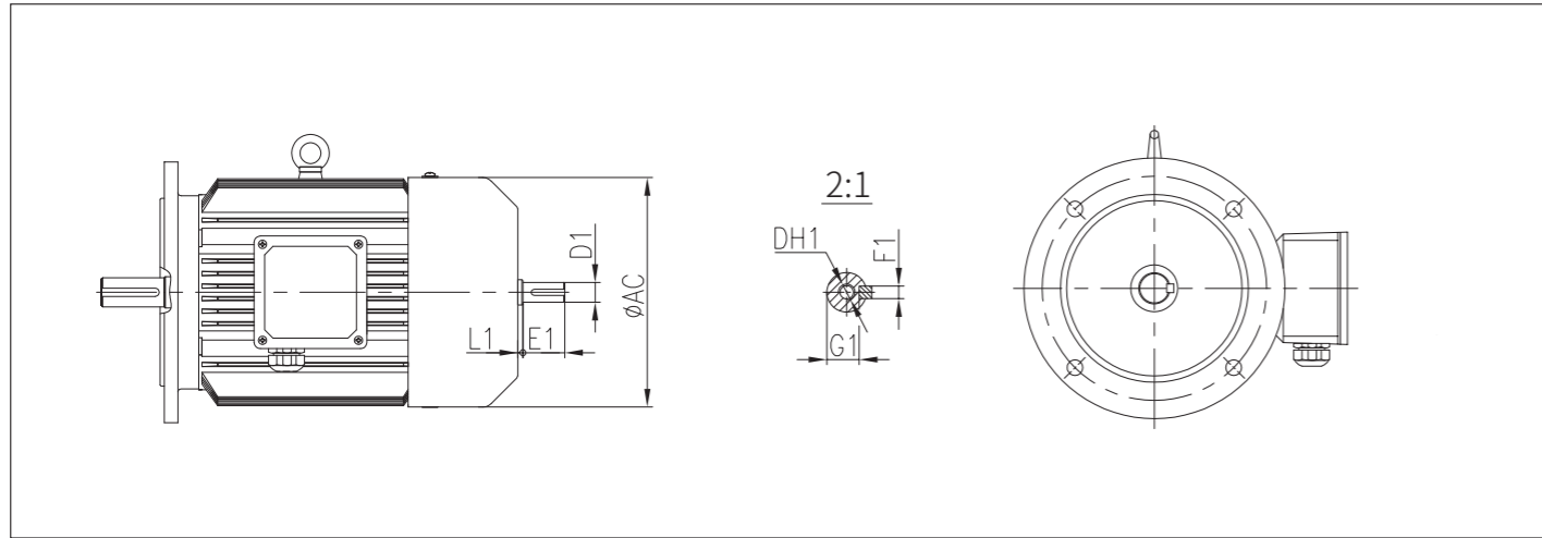
马达尾部出轴尺寸
