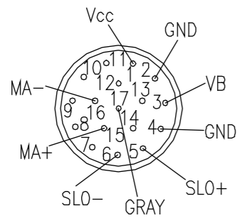
马达信号端插头 (Biss-C编码器) Motor signal end plug (Biss-C encoder)
