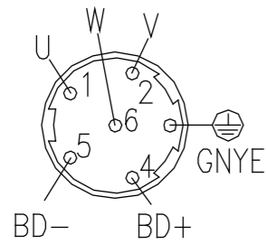
马达动力端插头 (28~80机座) Motor power end plug (28-80)
