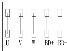
马达风机、制动器电气接线图 Motor fan & brake electrical wiring diagram
