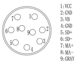
马达编码器接线图 Motor encoder wiring diagram
