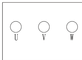
马达动力线接线图 Motor power line wiring diagram
