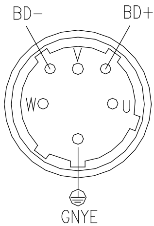
马达动力端插头 (100机座) Motor power end plug (100)
