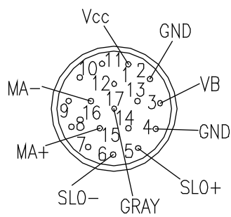
马达信号端插头 (Biss-C编码器) Motor signal end plug (Biss-C encoder)
