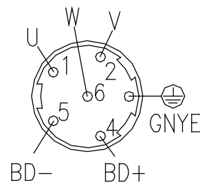
马达动力端插头 (28~80机座) Motor power end plug (28-80)
